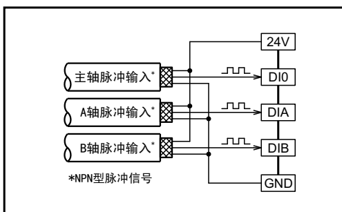
接近开关/编码器接线
