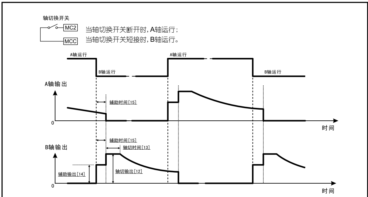
轴切换过程 - 收卷
